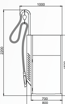
Combi BOY CB/T Combi BOY CAB/T
